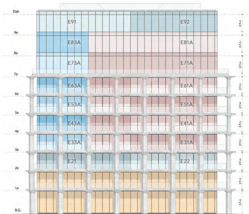
Pleinzijde: noord-west
