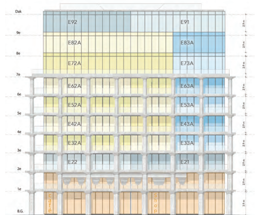
Singelzijde: zuid-oost
